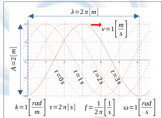
Figura 3: Onda coseno con ciertas características.
